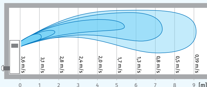
Zakres rozchodzenia się strumienia świeżego powietrza dla CIVIC EC LB 500 V.2
